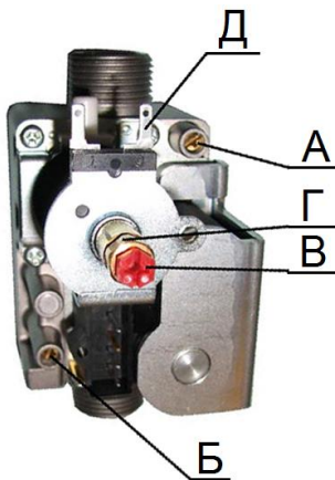
Рис. 9 Регулятор подачи газа
