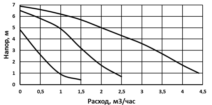
Рис. 13. Напорная характеристика насоса.
