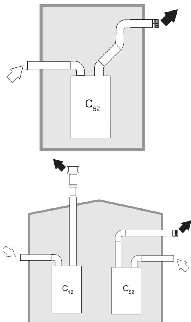
Рис. 4. Пример систем дымоудаления собранных с помощью отдельных труб. Белой стрелкой обозначен приток воздуха, черной стрелкой отвод продуктов сгорания
